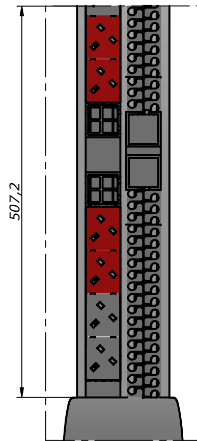
DETALLE A
